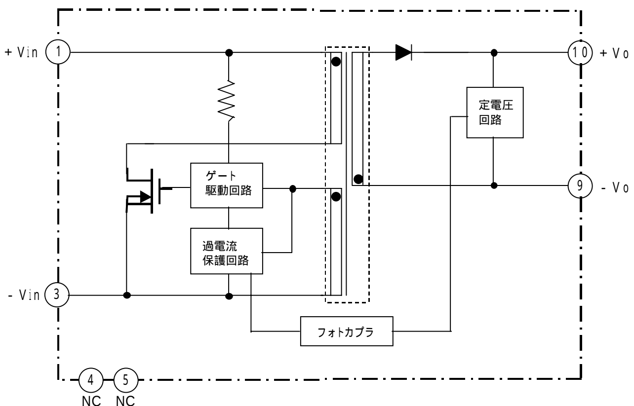
ブロック図
