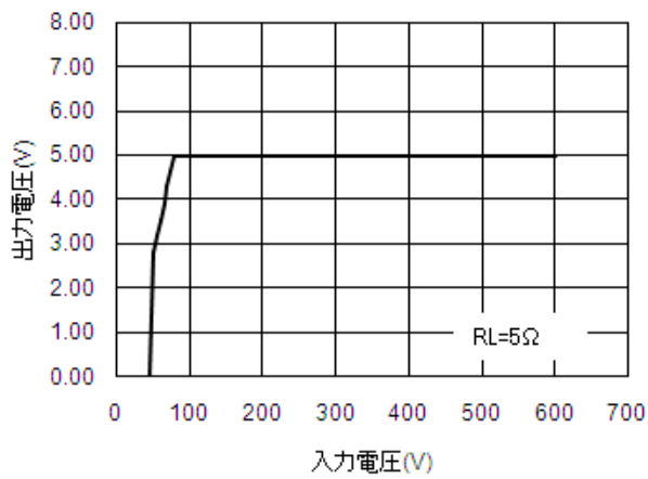
出力電圧-入力電圧特性
