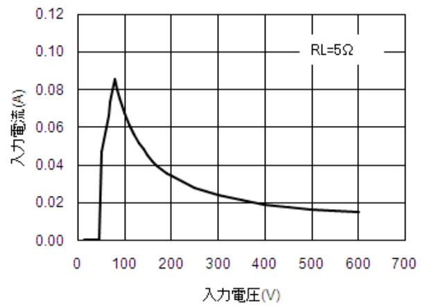
入力電流-入力電圧特性
