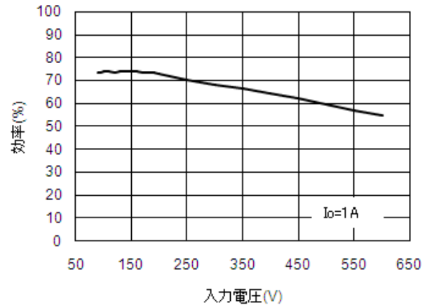
効率-入力電圧特性
