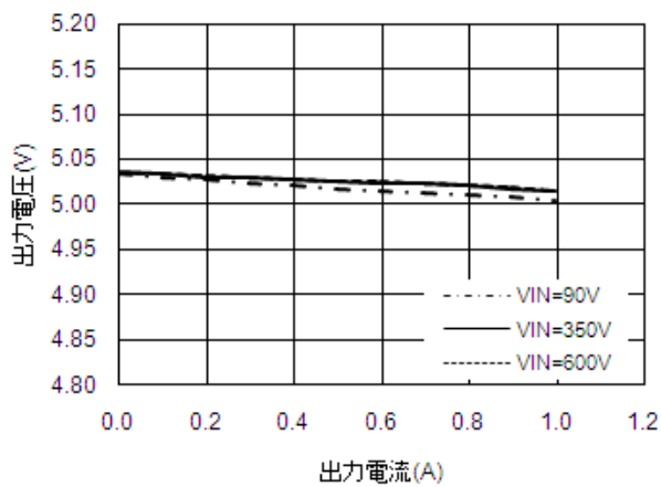
出力電圧-出力電流特性
