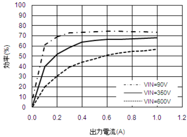
効率-出力電流特性
