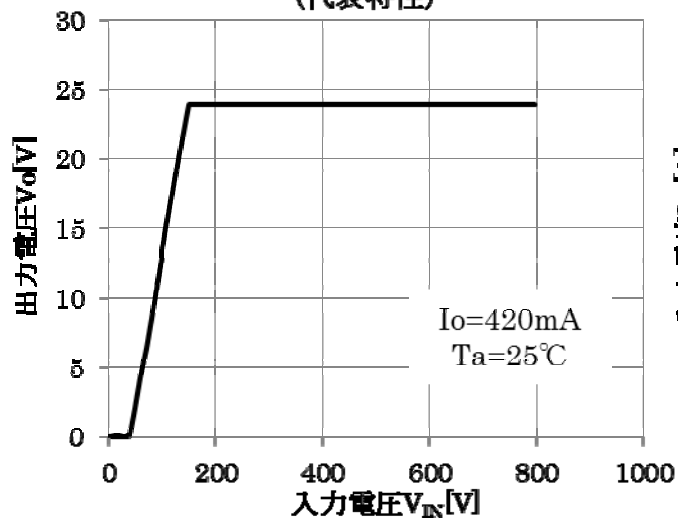
出力電圧-入力電圧特性 （代表特性）
