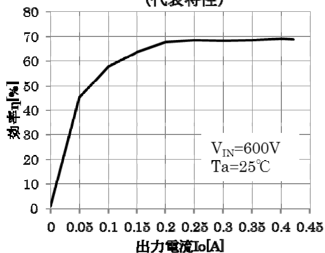
効率-出力電流特性 （代表特性）
