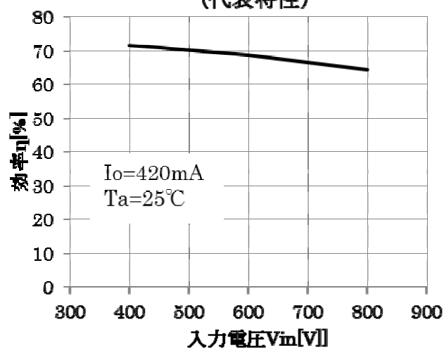
効率-入力電圧特性 （代表特性）
