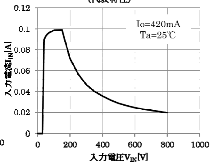
入力電流-入力電圧特性 （代表特性）
