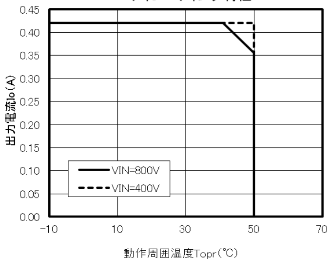
ディレーティング特性
