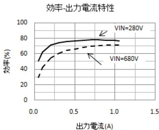
特性曲線 (代表例) T_a=25^{\circ}\text{C}
