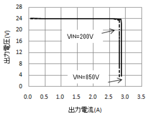
出力電圧-出力電流特性
