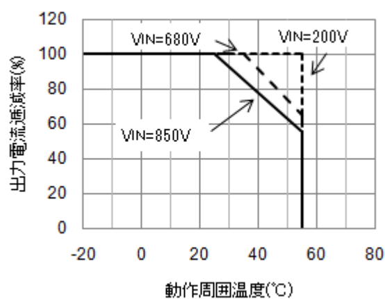
デレーティング特性
