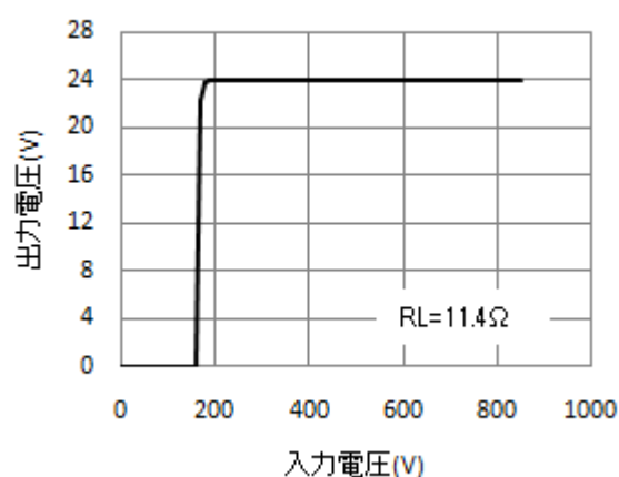
出力電圧-入力電圧特性
