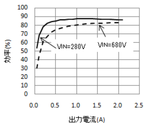
効率-出力電流特性
