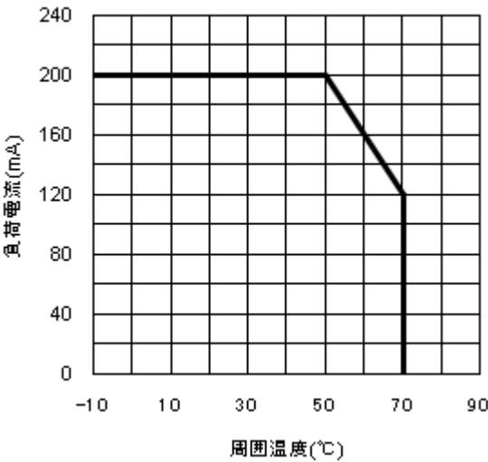
ディレーティング特性
