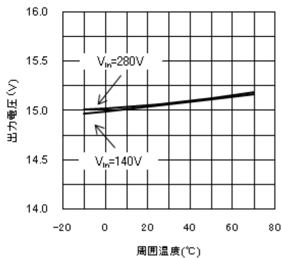
出力電圧-周囲温度特性
