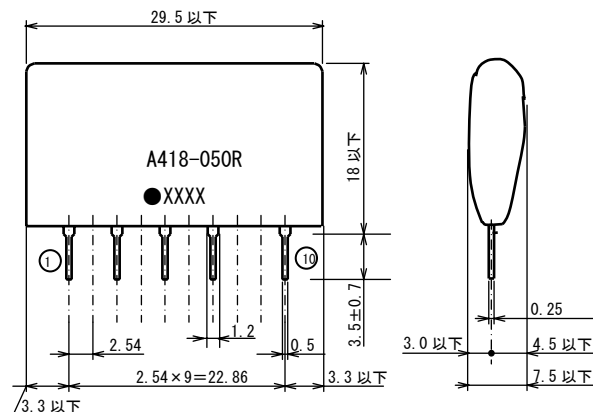
外形图
