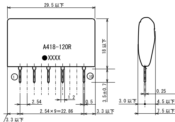
外形図
