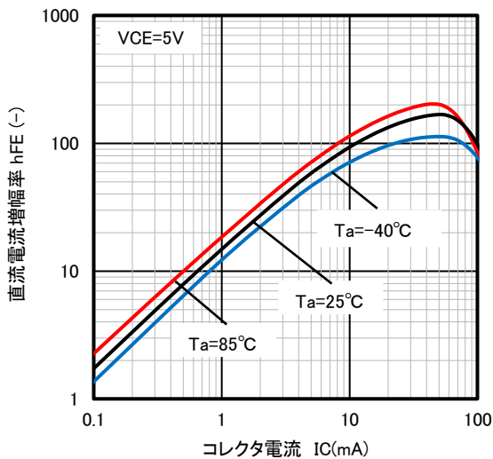
直流電流増幅率－コレクタ電流
