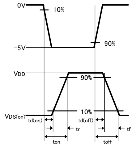
入力波形
