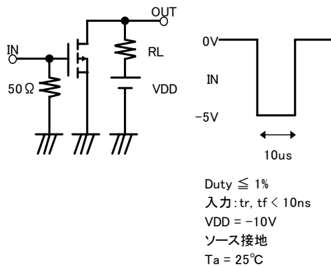
スイッチング時間測定回路
