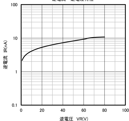
逆電流－逆電圧特性
