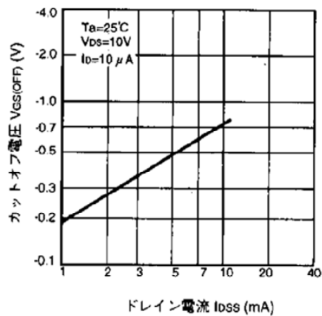
カットオフ電圧-ドレイン電流特性
