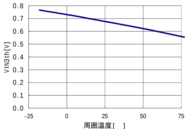
IN3閾値電圧 - 周囲温度特性
