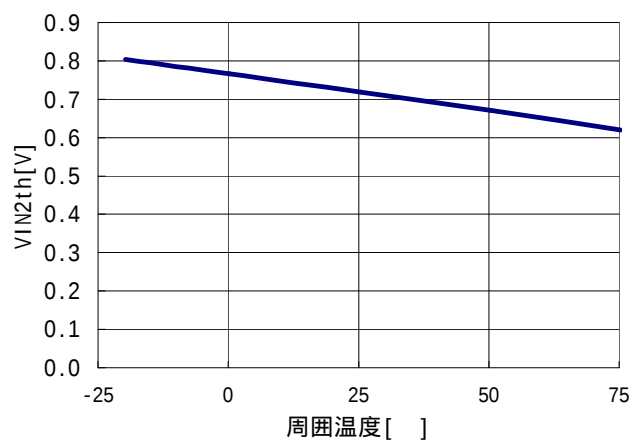
IN2閾値電圧 - 周囲温度特性
