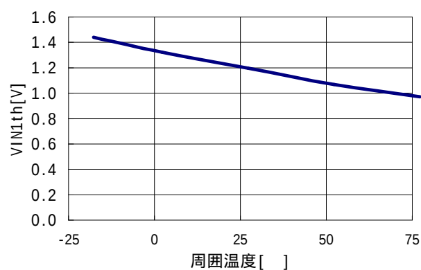
IN1閾値電圧 - 周囲温度特性
