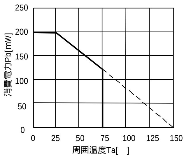
熱低減曲線
