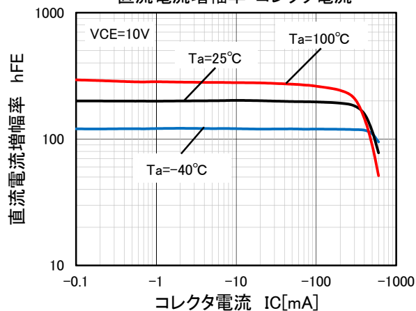
直流電流増幅率-コレクタ電流
