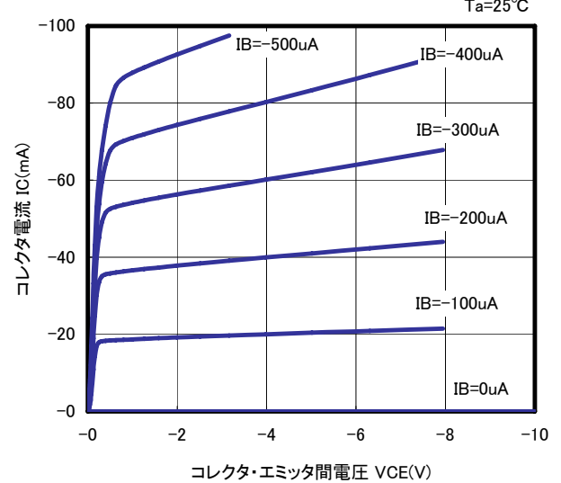
エミッタ接地出力特性
