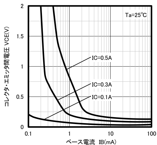
コレクタ・エミッタ間電圧 - ベース電流特性
