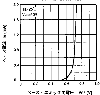
エミッタ接地入力特性
