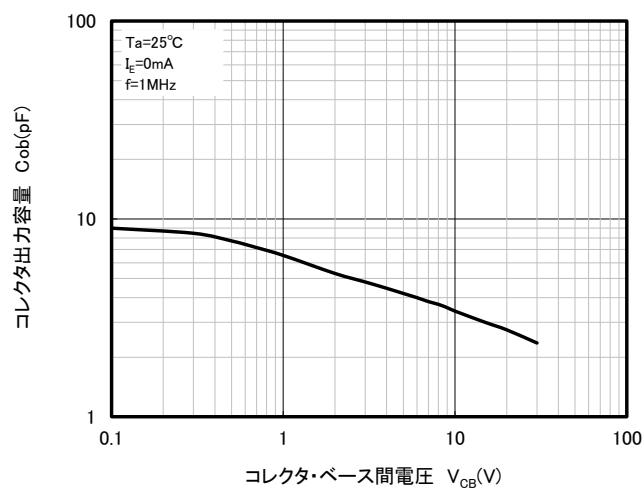
コレクタ出力容量－コレクタ・ベース間電圧
