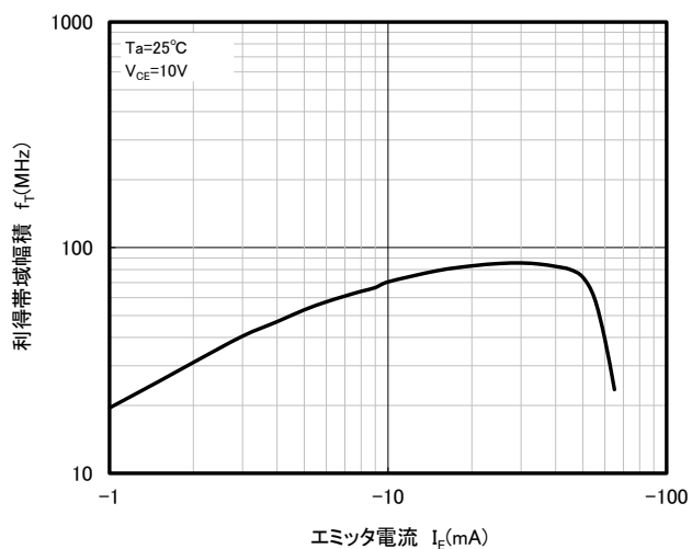
利得帯域幅積－エミッタ電流特性
