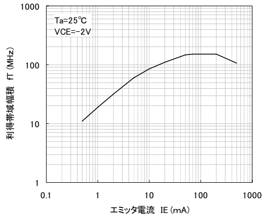
利得帯域幅積-エミッタ電流特性
