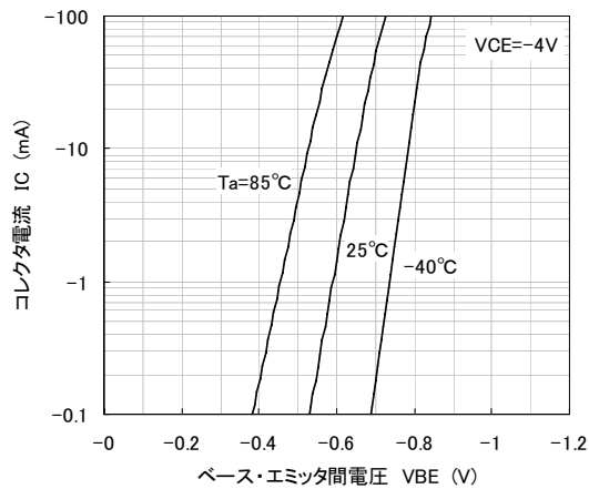
エミッタ接地伝達特性
