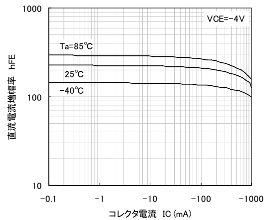
直流電流増幅率-コレクタ電流特性
