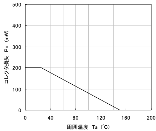
コレクタ損失-周囲温度特性
