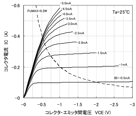
エミッタ接地出力特性
