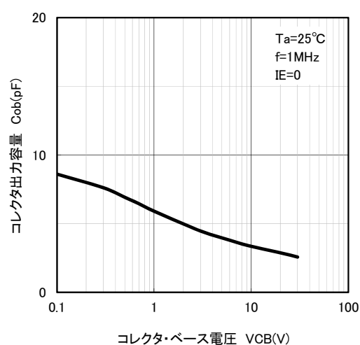
Cob-VCB特性グラフ
