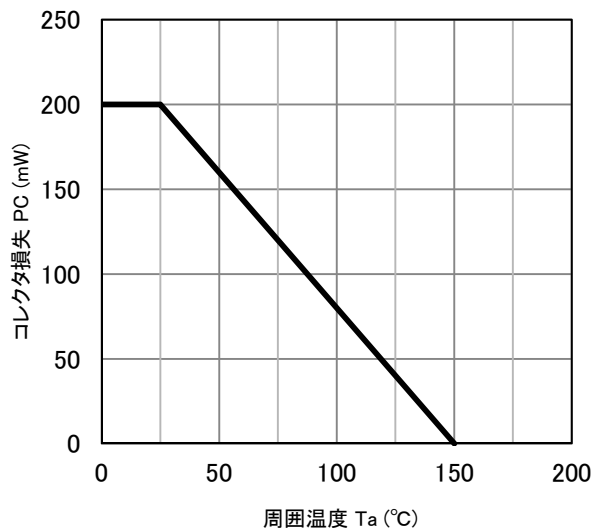
コレクタ損失-周囲温度特性
