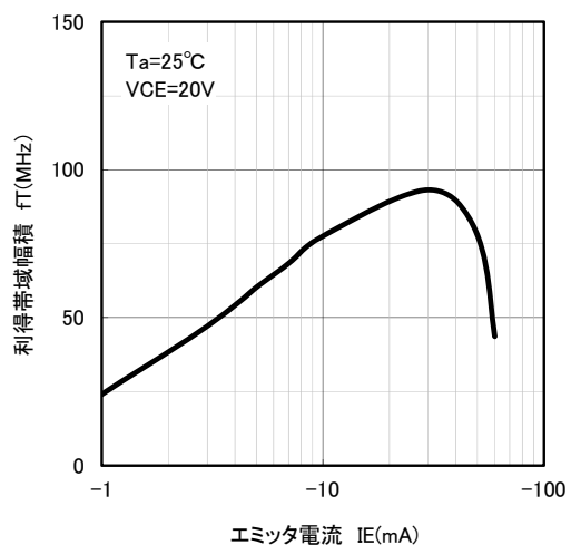
fT-IE特性グラフ
