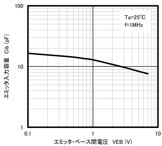
エミッタ入力容量-エミッタ・ベース間電圧特性
