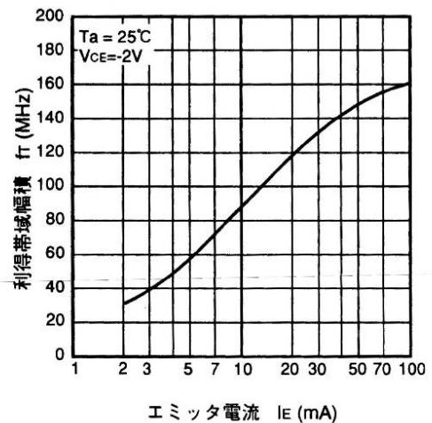
利得帯域増幅積-エミッタ電流特性
