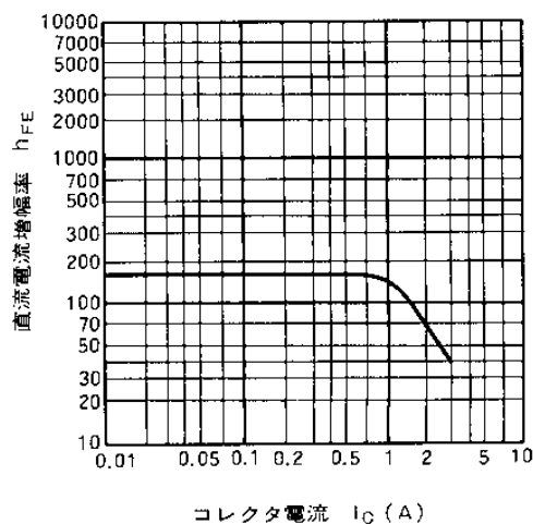
直流電流増幅率-コレクタ電流特性
