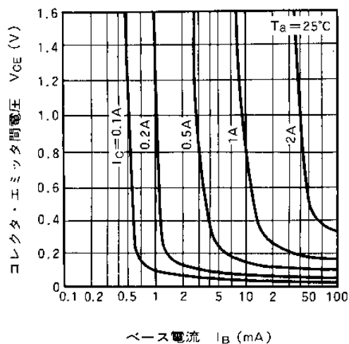
コレクタ・エミッタ飽和電圧- ベース電流特性
