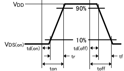
出力波形
