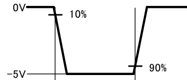
入力波形
