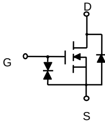
等価回路
