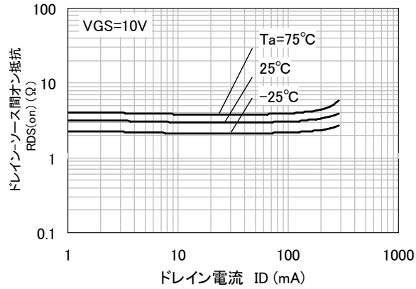
RDS(ON) - ID
