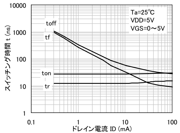
t - ID
