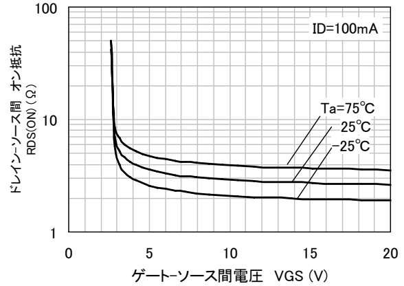
RDS(ON) - VGS
