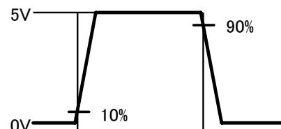
入力波形
