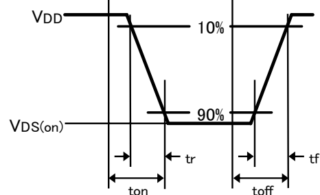
出力波形
