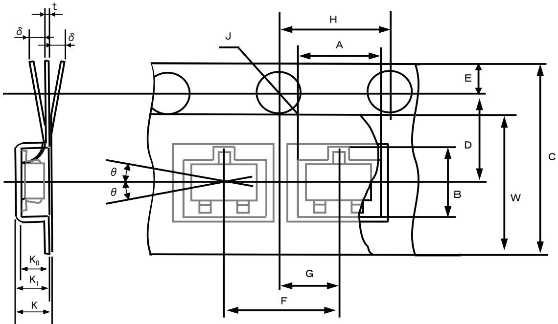
図1. テープ形状及び寸法
