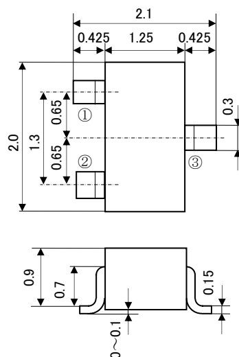
RT1P44BM
