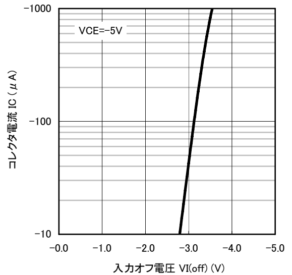
コレクタ電流－入力オフ電圧
