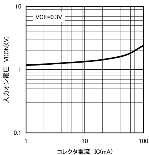
入力オン電圧－コレクタ電流
