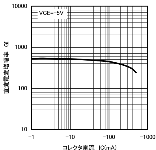
直流電流増幅率－コレクタ電流
