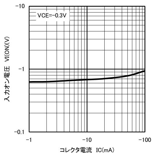
入力オン電圧－コレクタ電流
