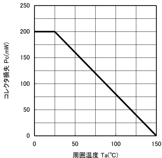
コレクタ損失－周囲温度特性
