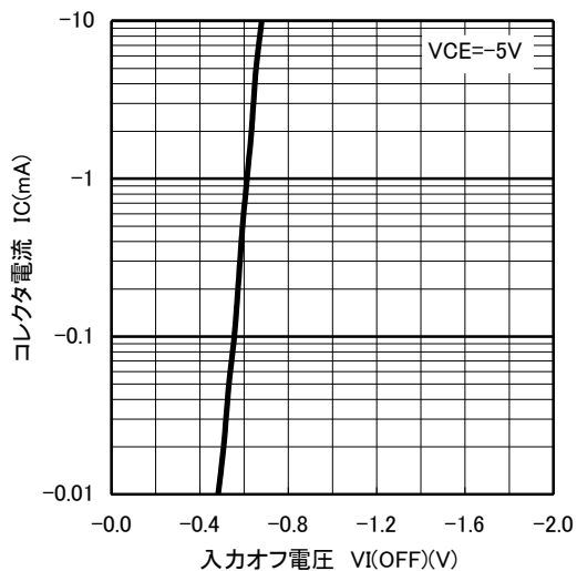
コレクタ電流－入力オフ電圧
