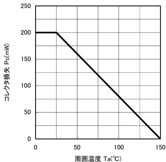
コレクタ損失－周囲温度特性
