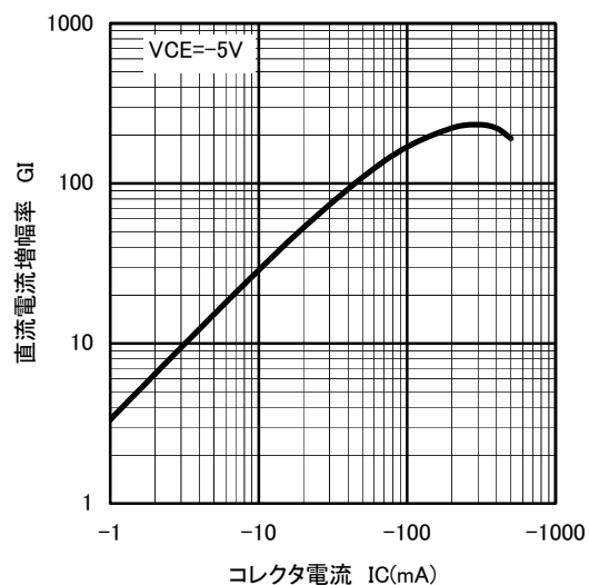
直流電流増幅率－コレクタ電流
