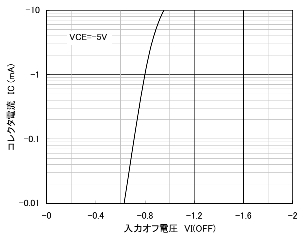
コレクタ電流-入力オフ電圧
