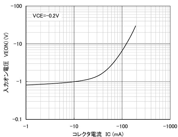
入力オン電圧-コレクタ電流
