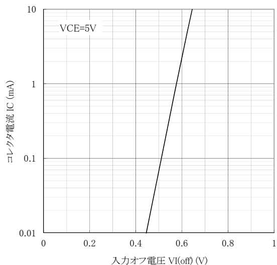
コレクタ電流 - 入力オフ電圧特性
