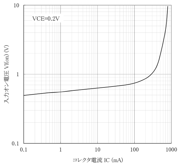
入力オン電圧 - コレクタ電流特性
