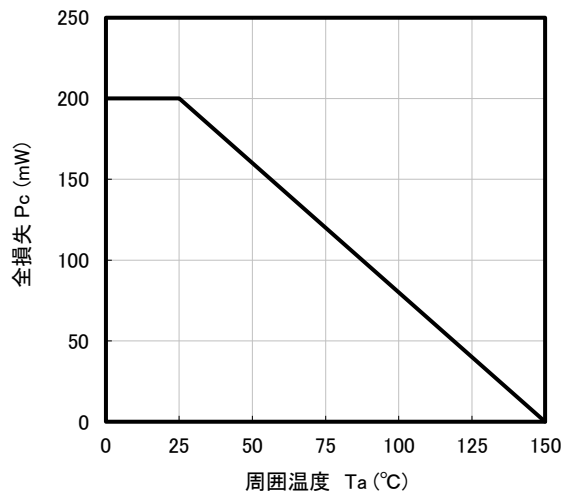
全損失-周囲温度特性
