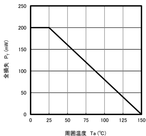
全損失-周囲温度特性
