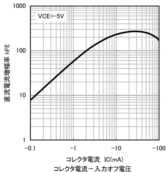
直流電流増幅率-コレクタ電流
