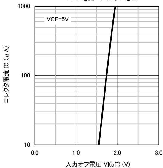
コレクタ電流-入力オフ電圧
