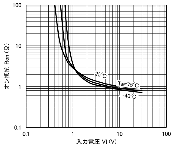
Ron-VI
