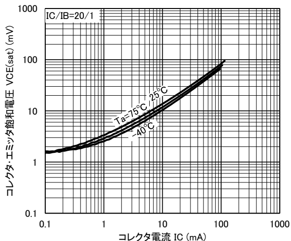
VCE(sat)-IC
