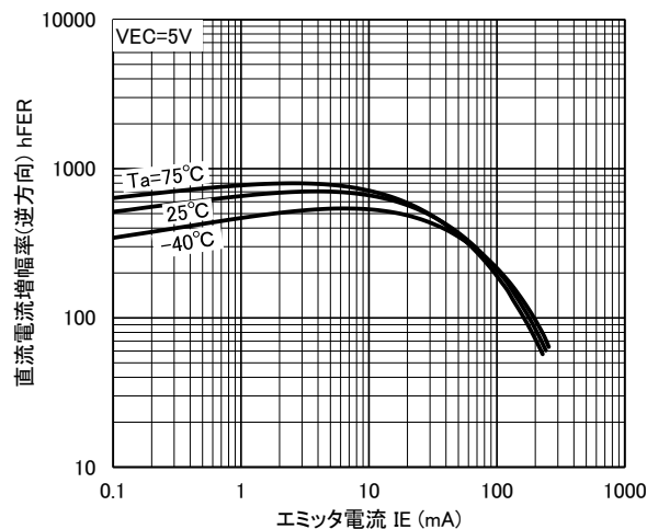
hFER-IE
