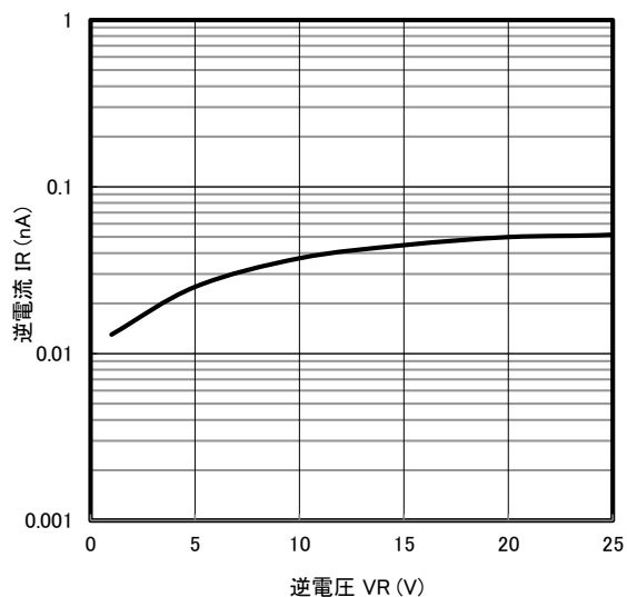
逆電流－逆電圧特性
