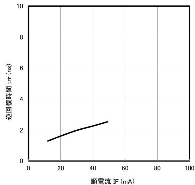
逆回復時間－順電流特性
