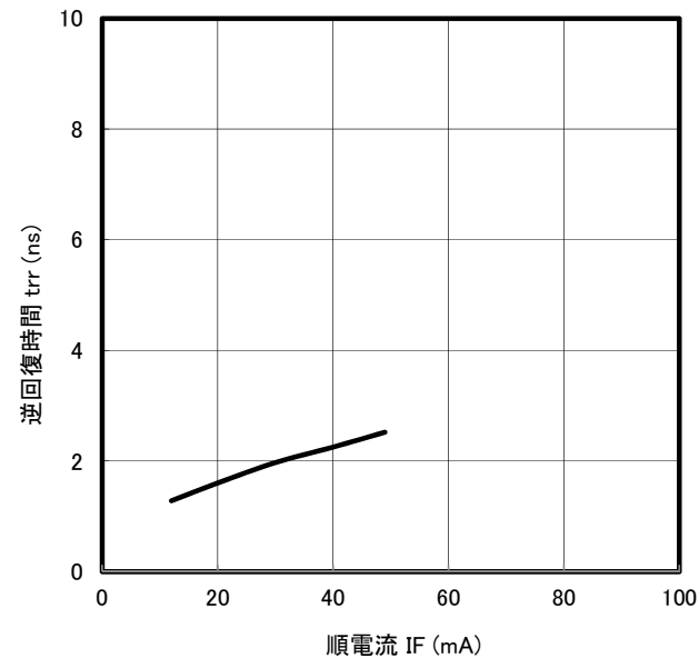
逆回復時間－順電流特性
