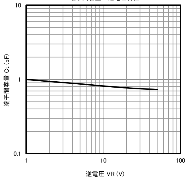
端子間容量－逆電圧特性
