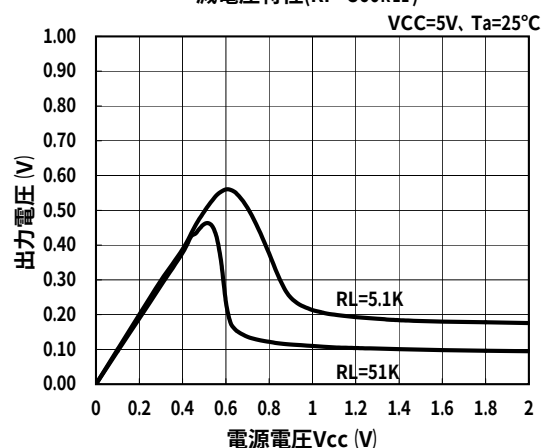
減電圧特性(RP=360kΩ)
