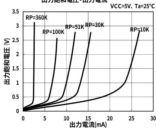
出力飽和電圧-出力電流
