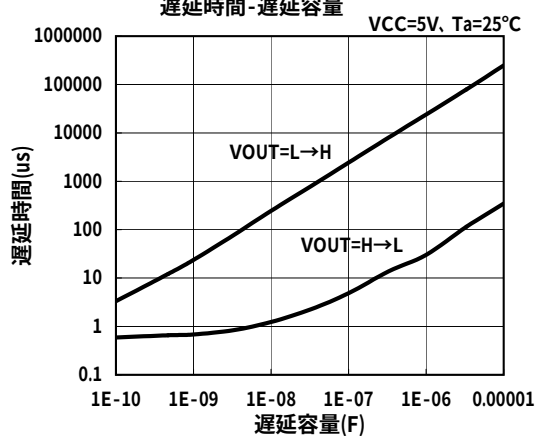
遅延時間-遅延容量
