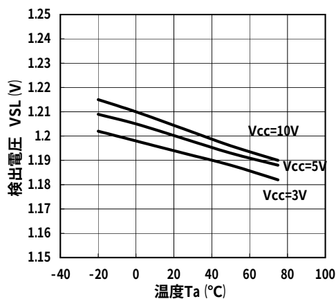
検出電圧-温度特性
