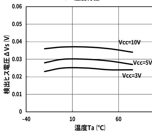
\Delta V_s -温度特性
