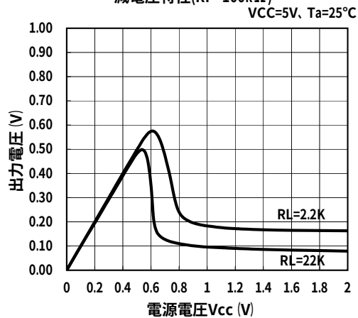
減電圧特性(RP=100kΩ)
