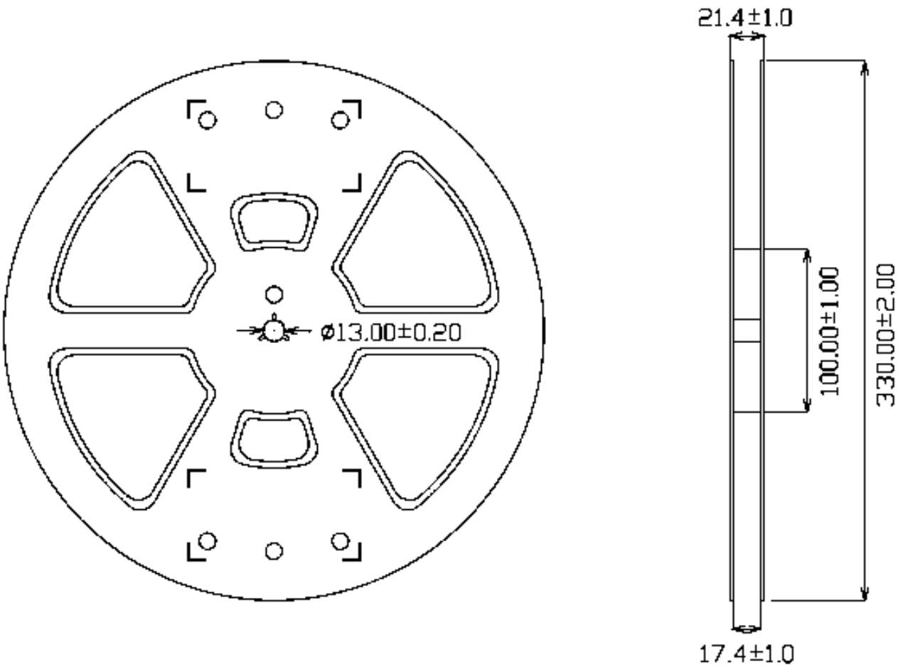
図2. リール形状及び寸法
