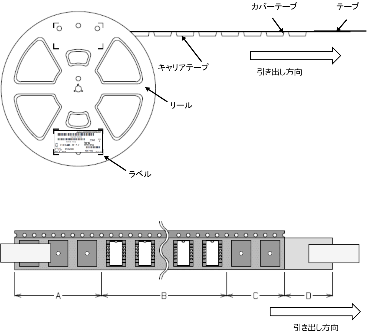
図3. リーダおよびトレイラ部仕様
