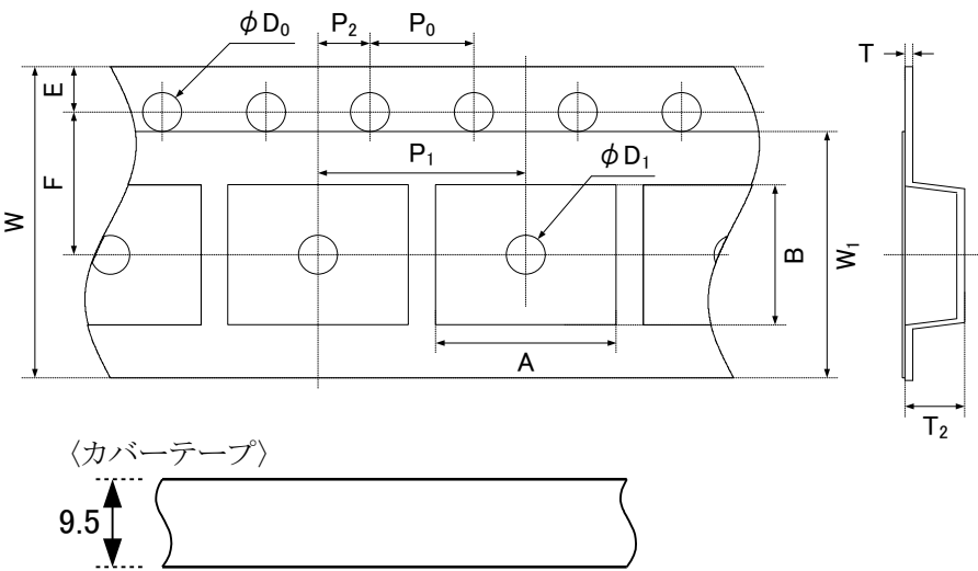
図1. テープ形状及び寸法
