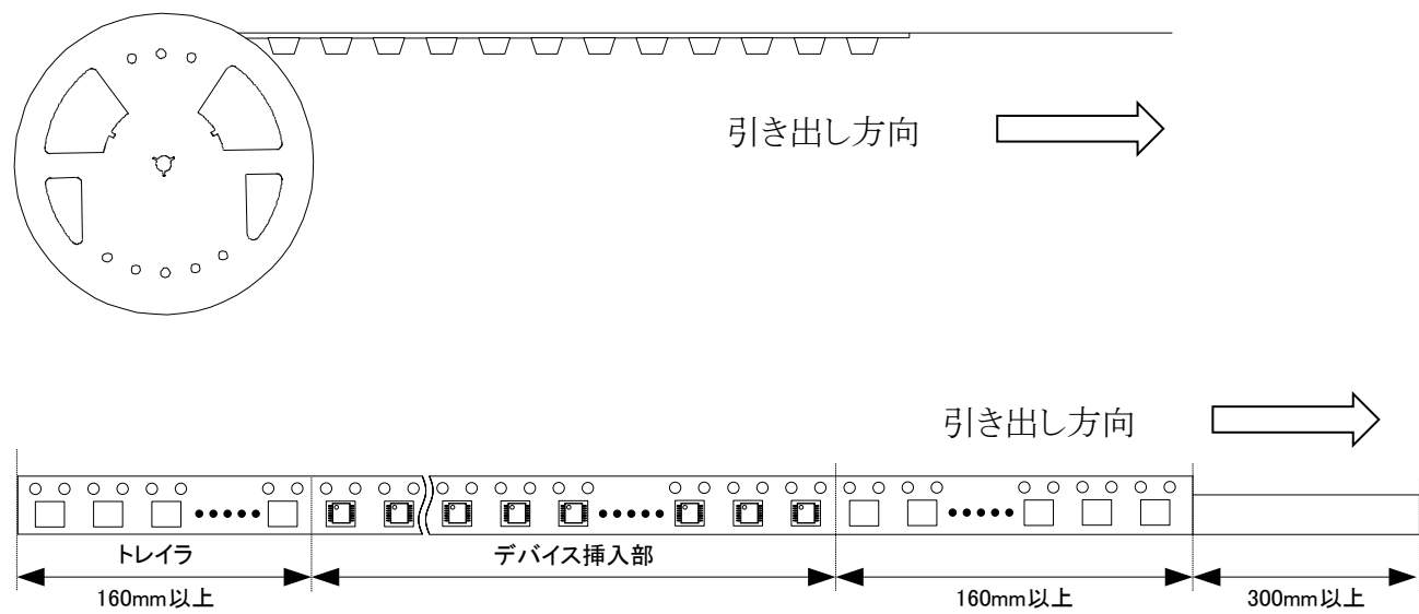
図3. リーダおよびトレイラ部仕様
