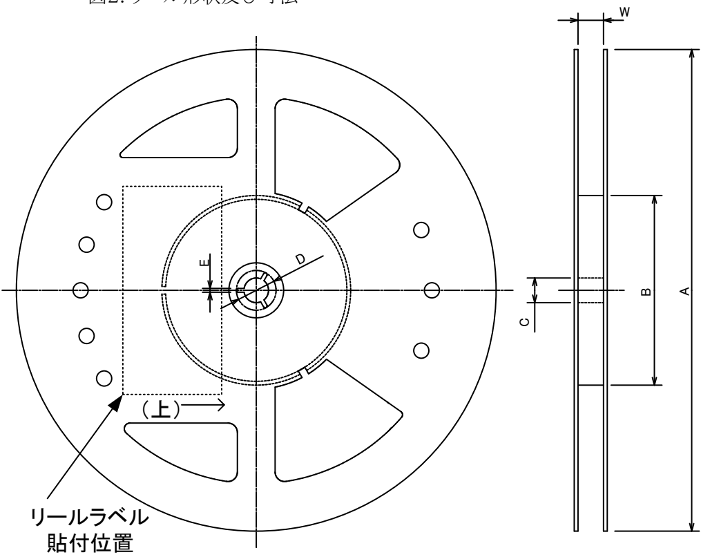
図2. リール形状及び寸法
